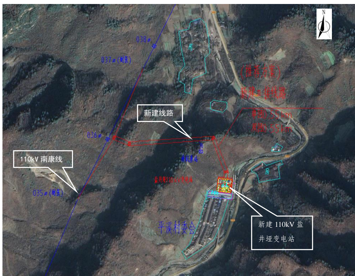
图 2.1-1 项目地理位置及线路走向图
