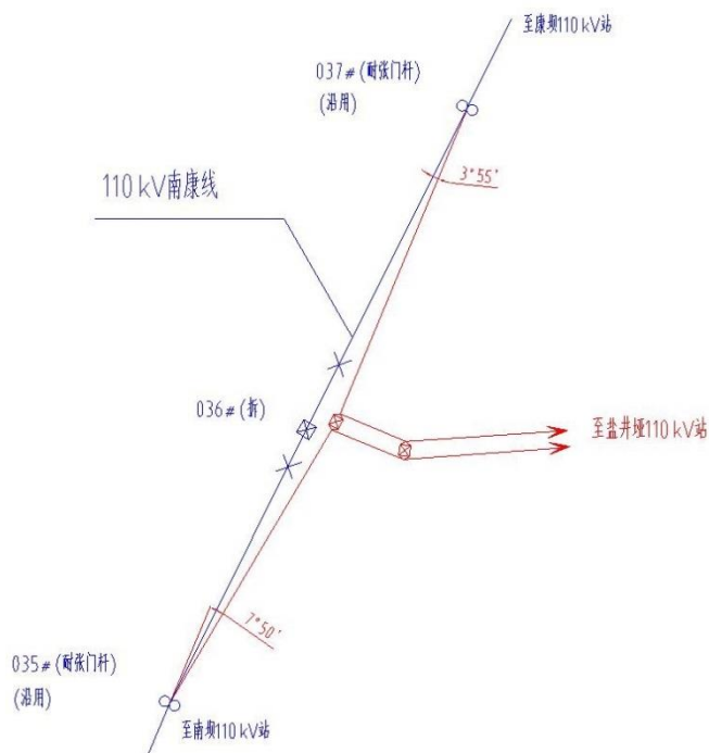
图 2.1-2 拆除线路工程
